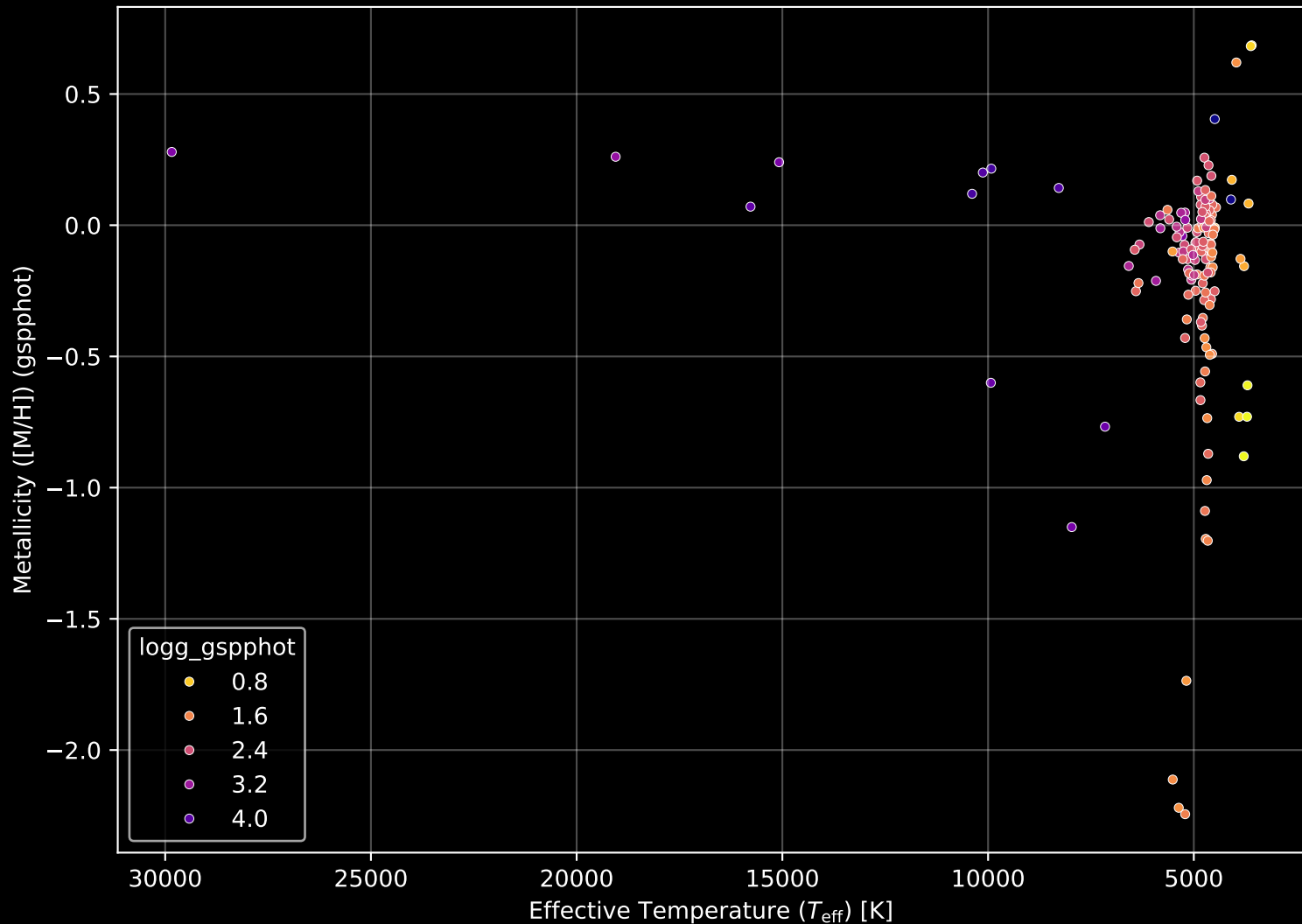
APOGEE DR17 Field: [Cas_N] Stellar Population Parameters (n= 145)
